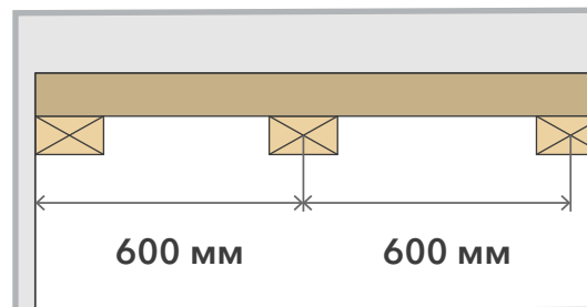
Каркас из деревянного бруска.
