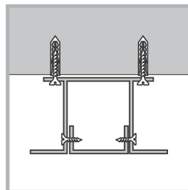
Профиль крепим на подвесы.
